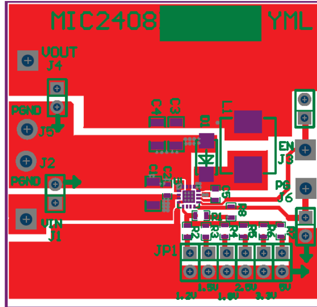
Top Layer
